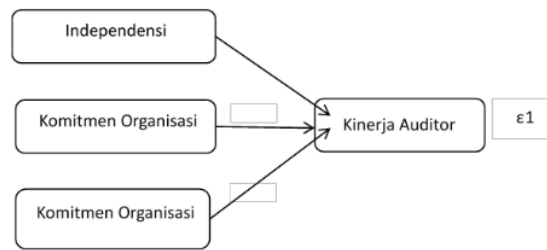
Gambar 1. Kerangka Konseptual
